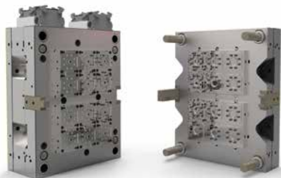
Spritzgießwerkzeug
