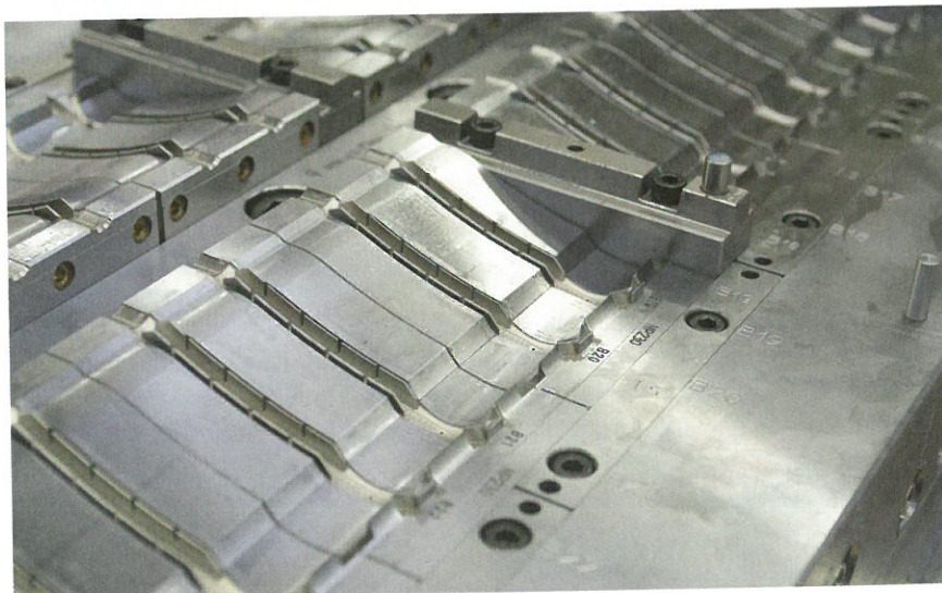
Kompetenz für Multikavitäten: ein Beispiel für Mehrkomponenten-Spritzgießwerkzeuge aus dem Hause Braunform. (© Heidenhain)
